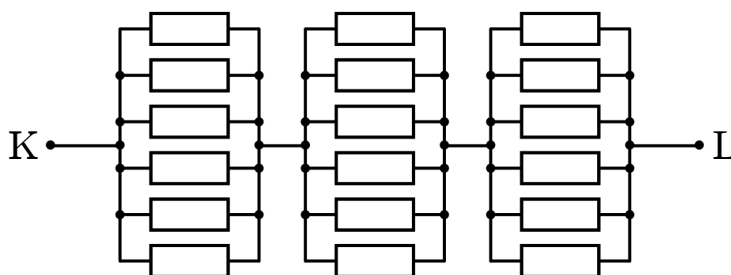
Obr. 1: Schéma zapojenia
